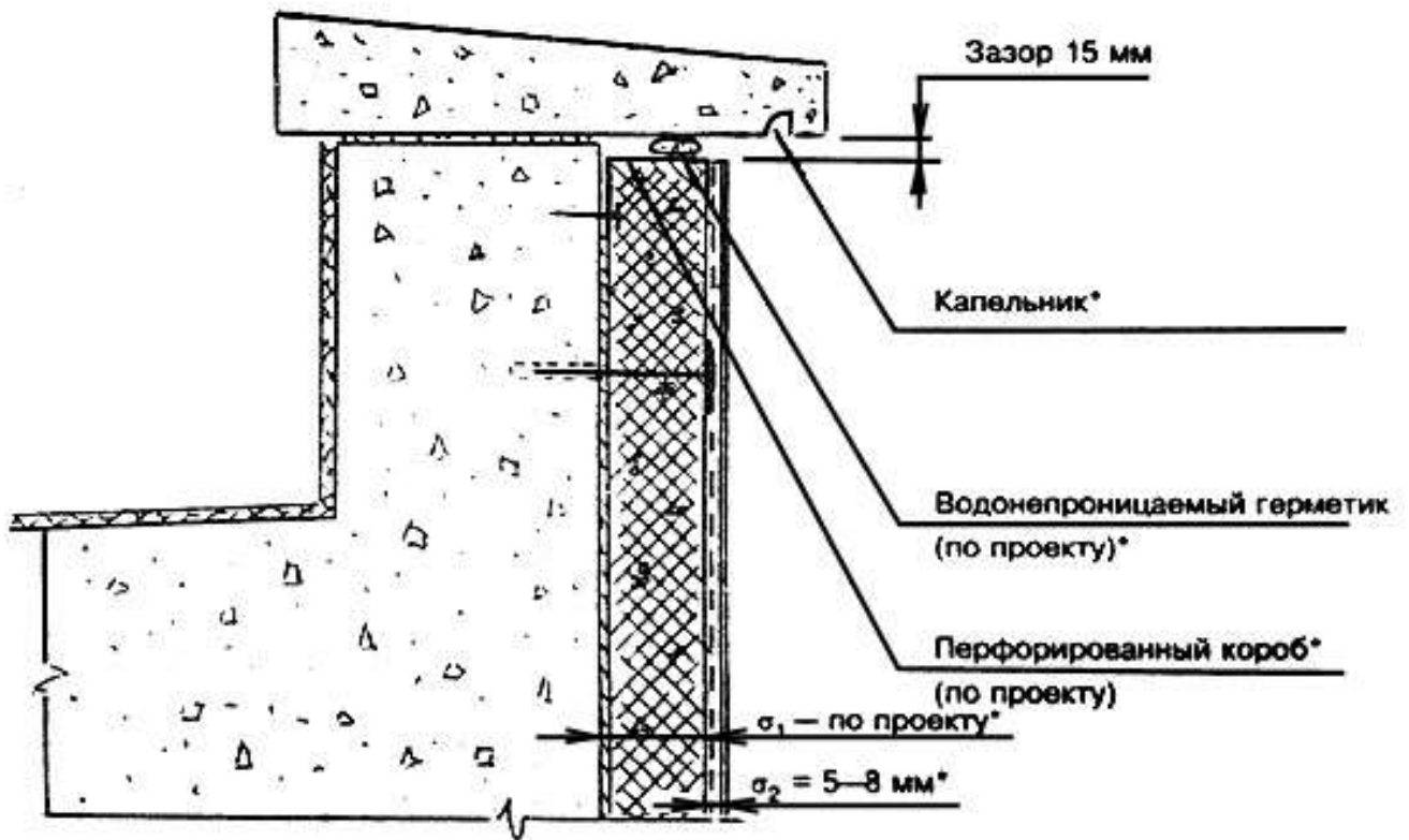
Рисунок 11. Фрагмент примыкания наружной теплоизоляции здания к карнизной плите
