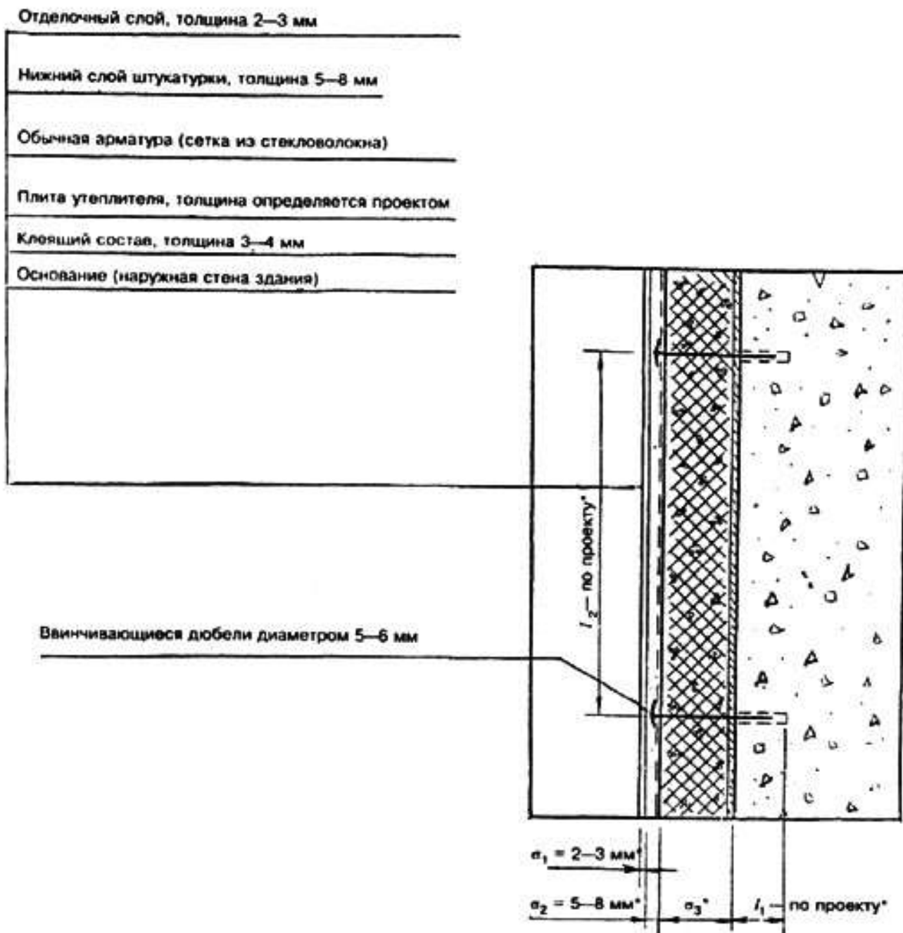
Рисунок 1. Фрагмент наружной теплоизоляции здания с тонкой штукатуркой по утеплителю
