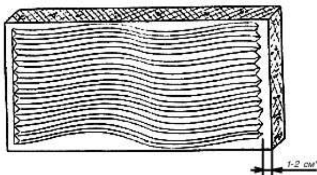
Рисунок 5. Сплошной способ нанесения клеящего состава на поверхность плит утеплителя
