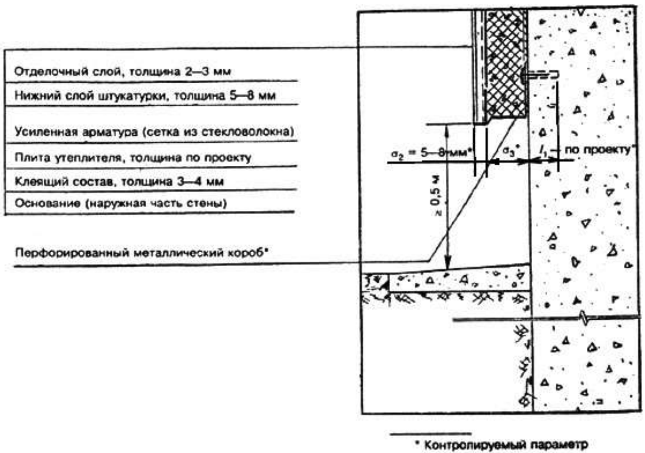
Рисунок 8. Крепление теплоизоляционного слоя на нижней части стены
