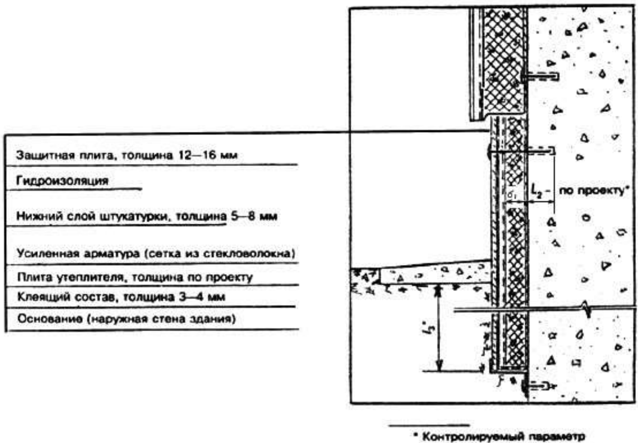
Рисунок 9. Фрагмент утепления нижней (и ее заглубленной) части стены здания
