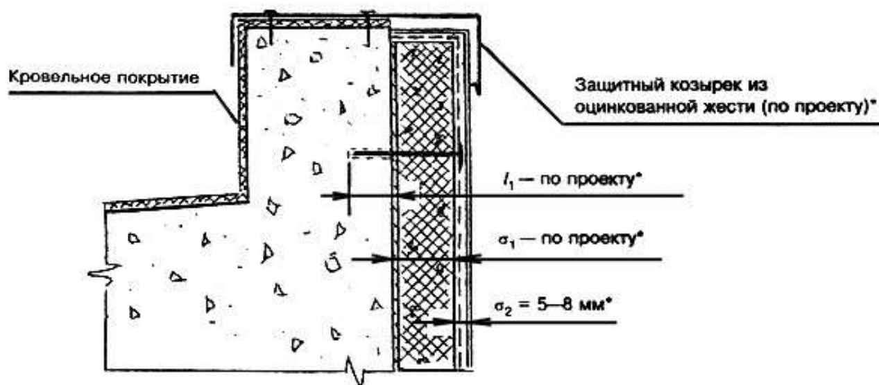
Рисунок 10. Примыкание теплоизоляционного слоя к парапету в верхней части фасада
