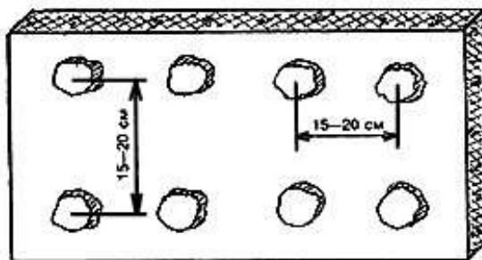
Рисунок 3. Маячковый способ нанесения клеящего состава на поверхность плит утеплителя
